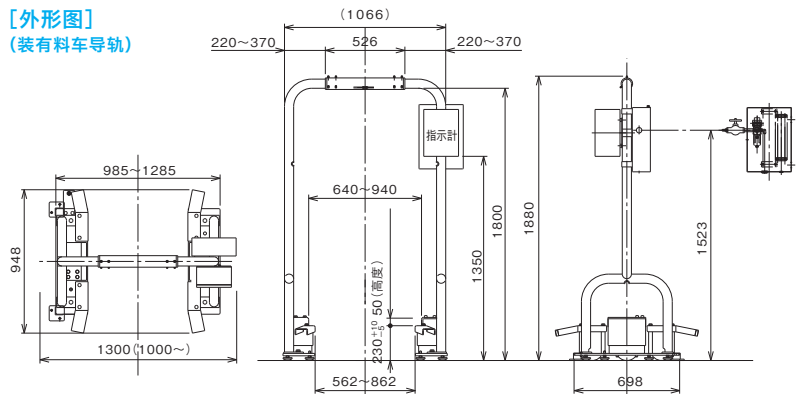
久田的重量指示计 (FC-W)
