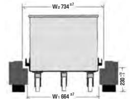
可适用料车的尺寸
