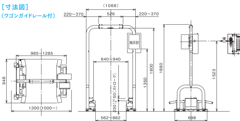
クボタの重量指示計(FC-W)
